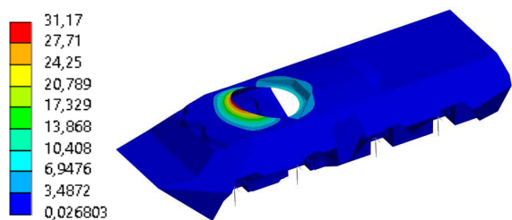
Картини розподілу повних переміщень, мм
