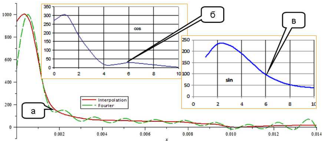
Рисунок 2 – Розподіл сили ударно-імпульсної взаємодії F_{\text{имп}}(t) (кН) між вибивною машиною і технологічним вантажем на інтервалі ненульового значення (15 мс) та її подання у вигляді частинної суми ряду Фур'є (див. формулу (1)):
