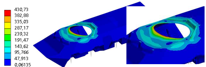
Картини розподілу еквівалентних напружень, МПа
