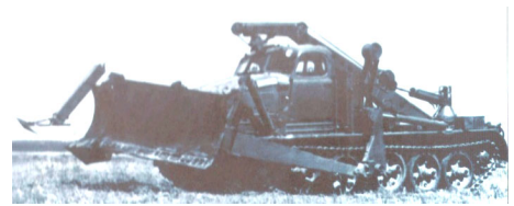
БАТ-М на базі виробу 405 МУ
