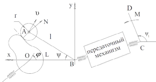
Рисунок 1 – Обобщенная схема механизма с кулачком [11]
