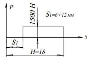
Рис. 4 – Зависимость силы P (см. рис. 3) от перемещения ползуна
